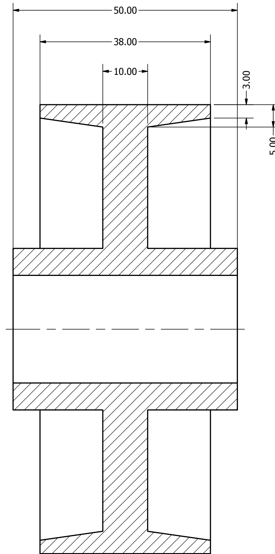
SECTION A-A SCALE 2:1
